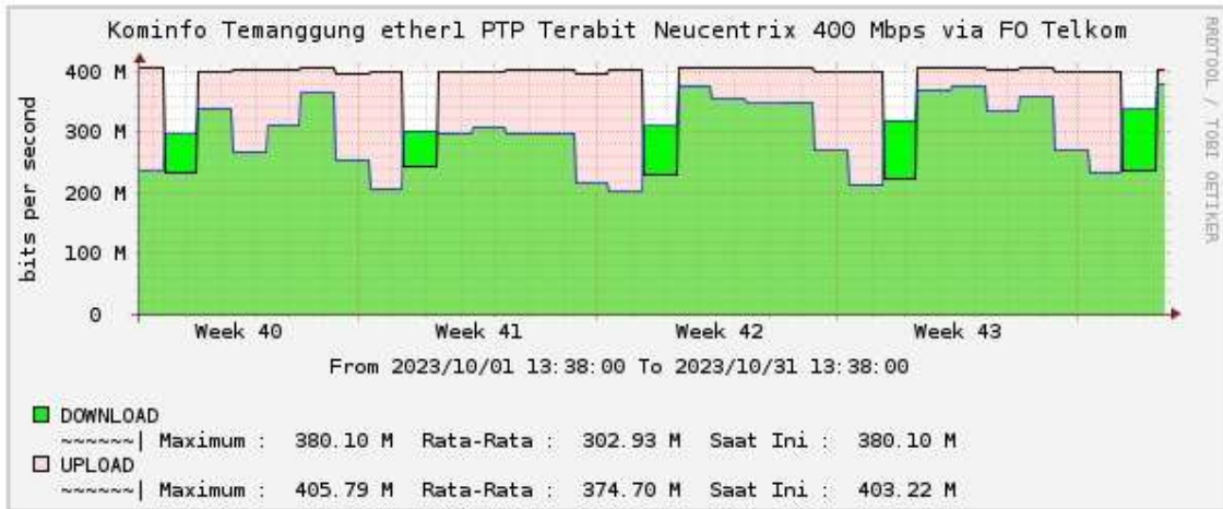
01-31 Oktober 2023 Via Telkom
