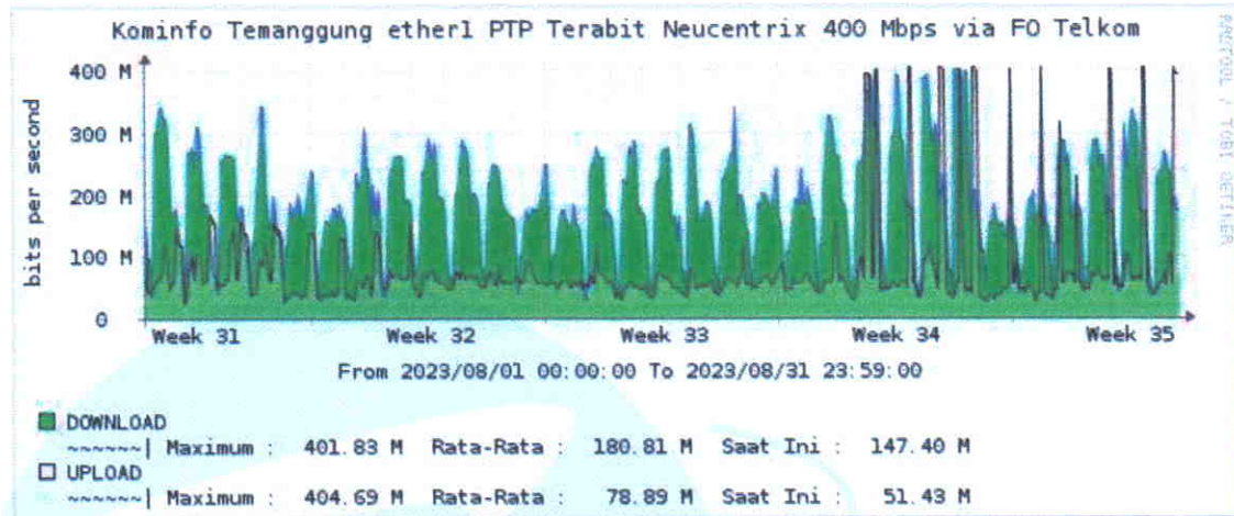
Kominfo Temanggung ether1 PTP Terabit Neucentrix 400 Mbps via FO Telkom
